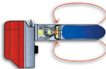
Einstufiger Blaubrenner mit LPC*-Technik
